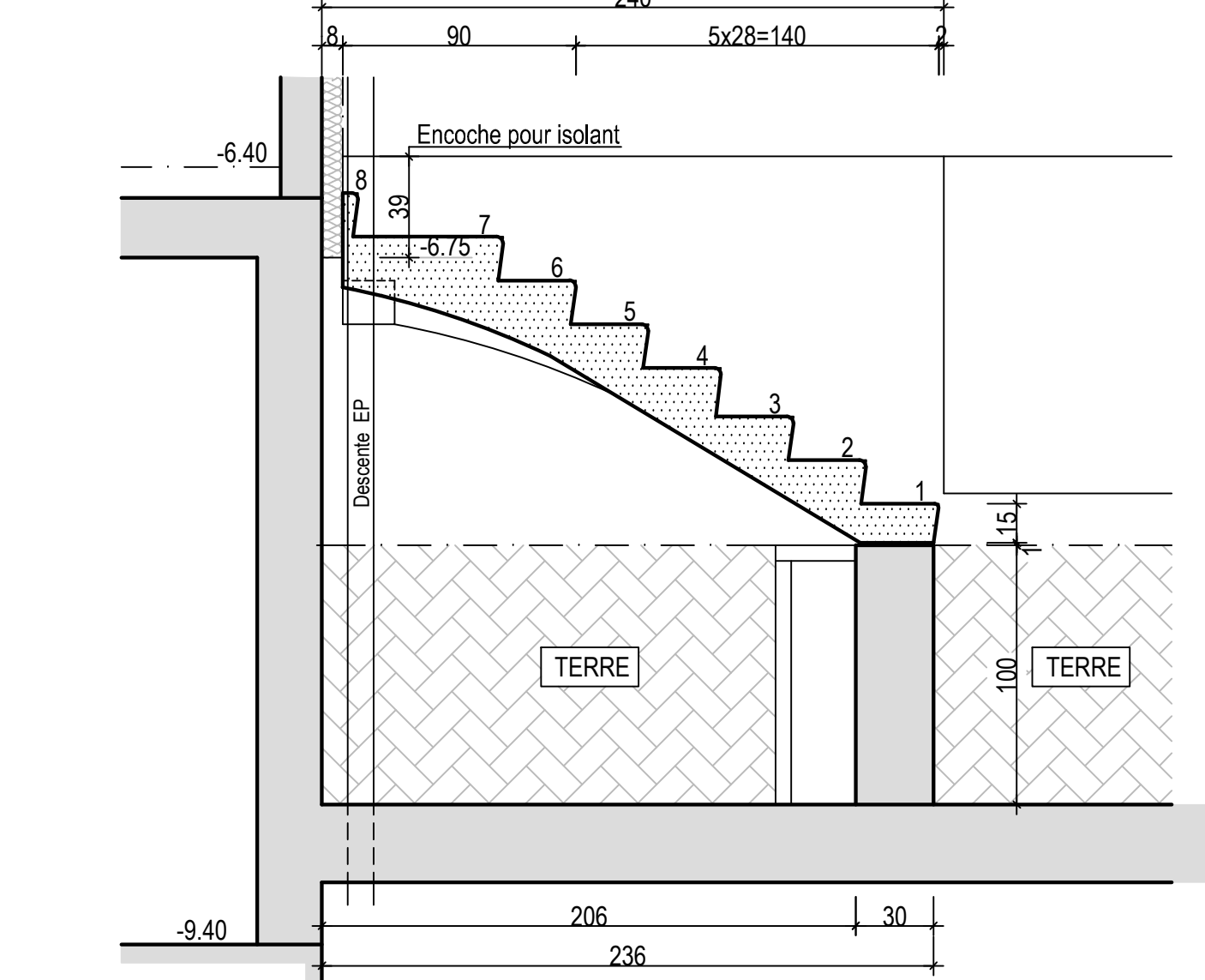
COUPE H
