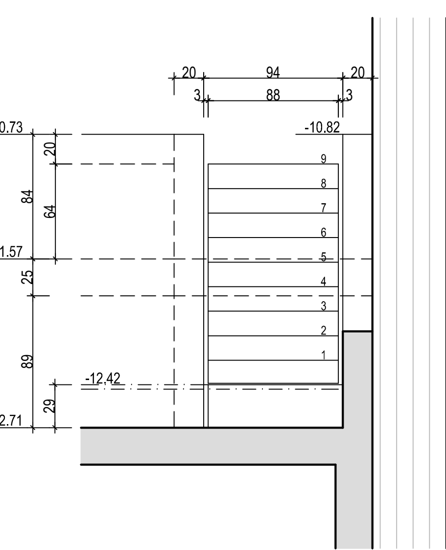
COUPE D
