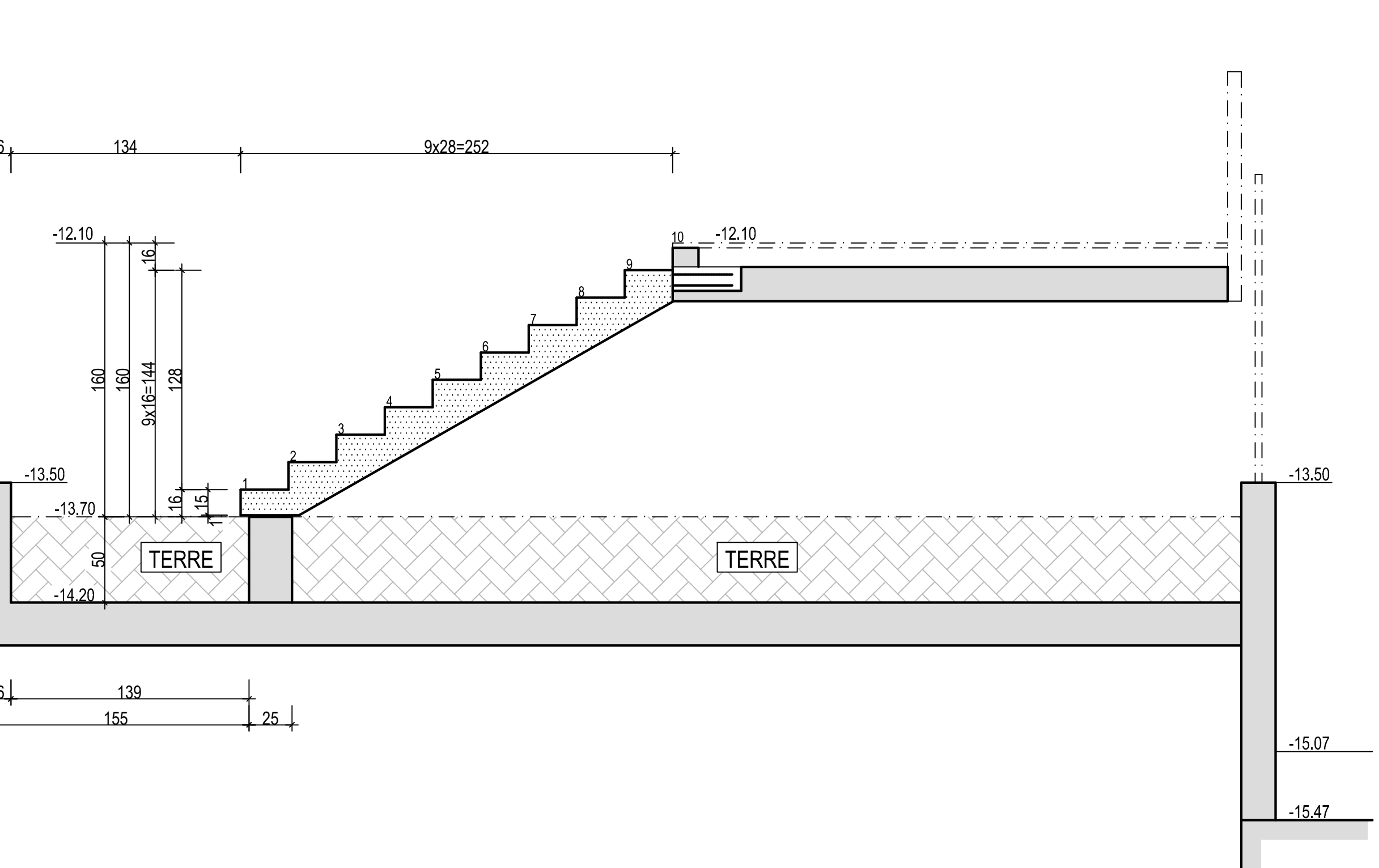
COUPE A
