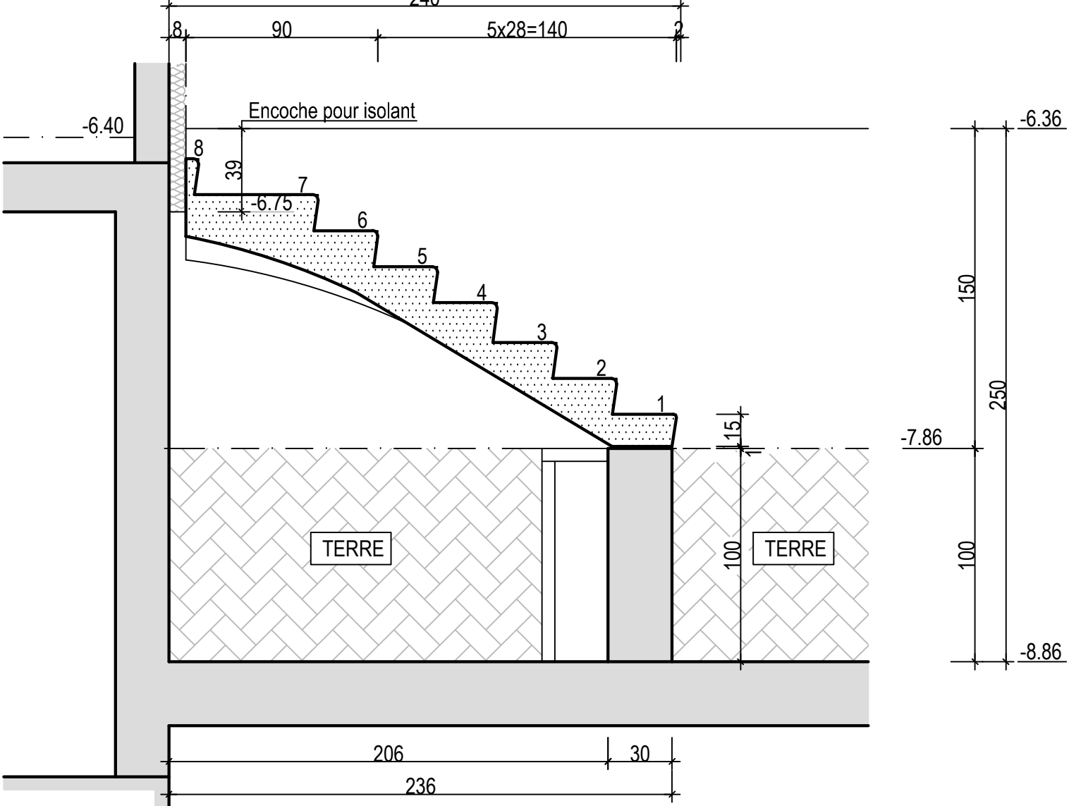
COUPE F
