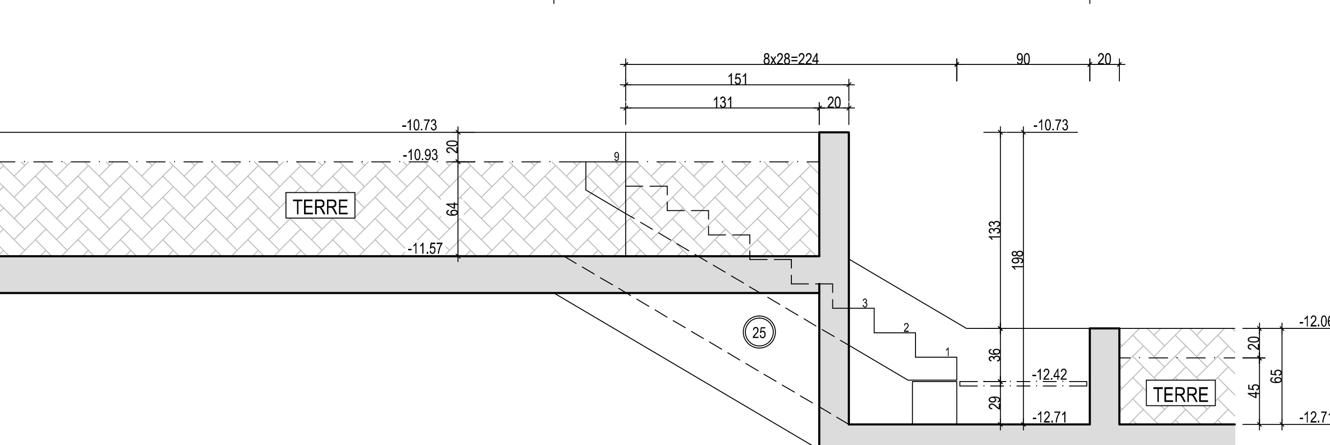
COUPE C
