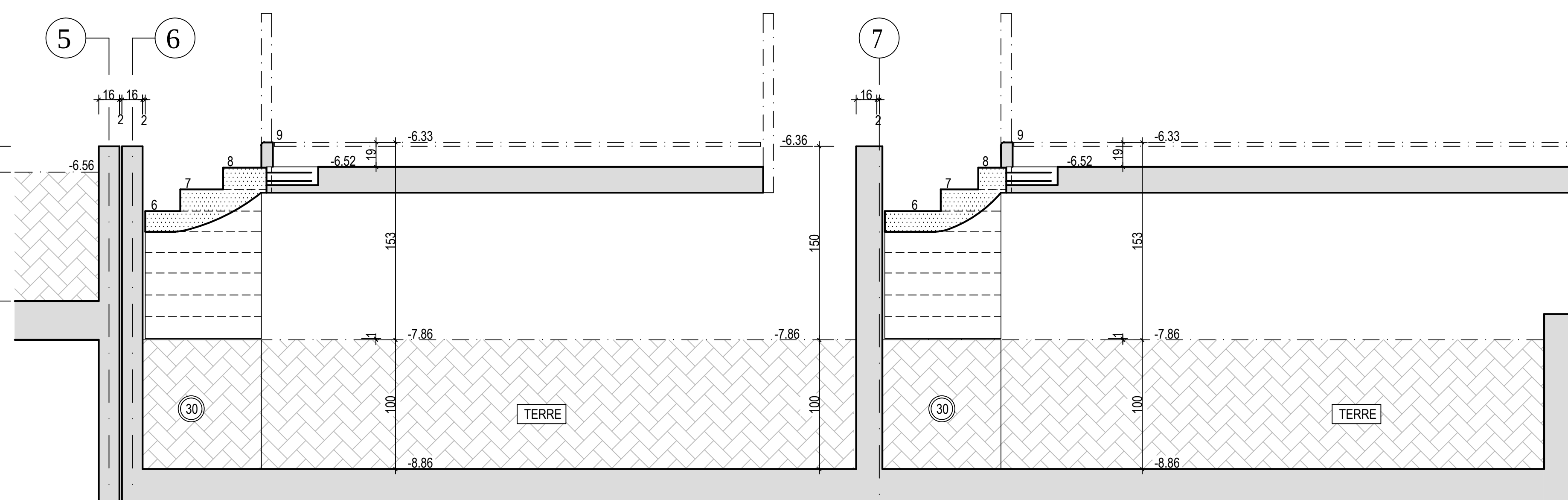
COUPE H
