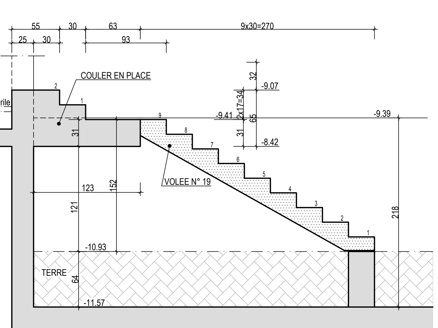
COUPE E
